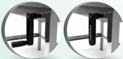
Manovella di comando regolazione altezza Height adjustable crank command
